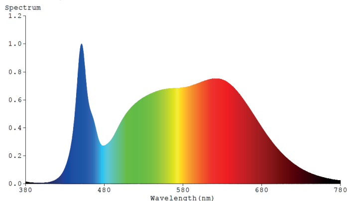
Spektrální graf DC24-4000K
